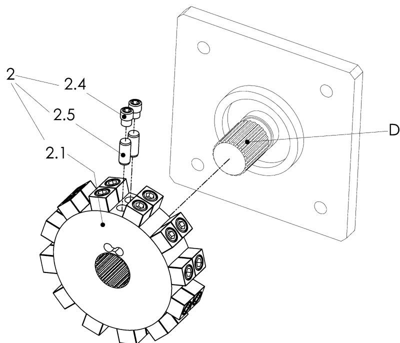
Abbildung 5-5 Nabenstern (2) mit CENTALOC-Klemmung montieren
