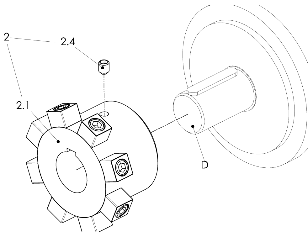
Abbildung 5-3 Nabenstern (2) mit zylindrischer Bohrung und Passfedernut montieren
