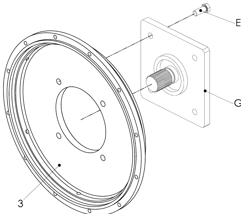
Abbildung 5-2 Adapter montieren
