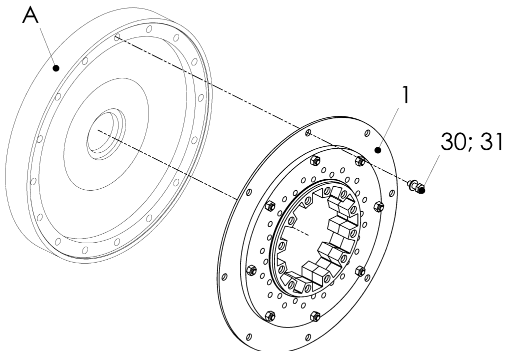
Abbildung 5-1 Elastikelement (1) montieren
