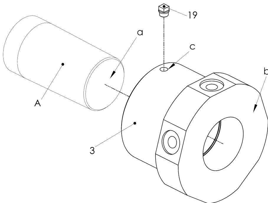
Abbildung 6-4 Nabe mit kegeligem Ölpressverband montieren
