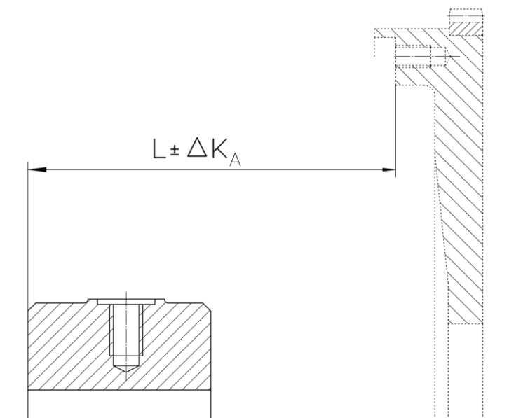
Abbildung 5-1 Axialer Ausrichtversatz
