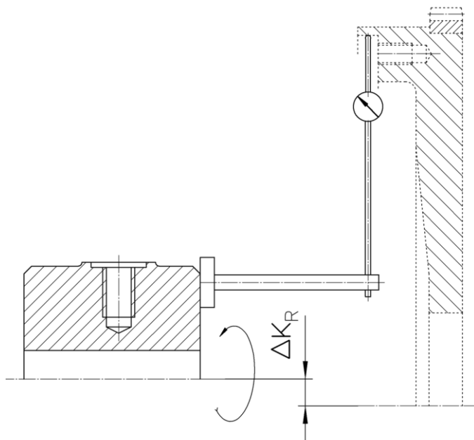
Abbildung 5-2 Radialer Ausrichtversatz
