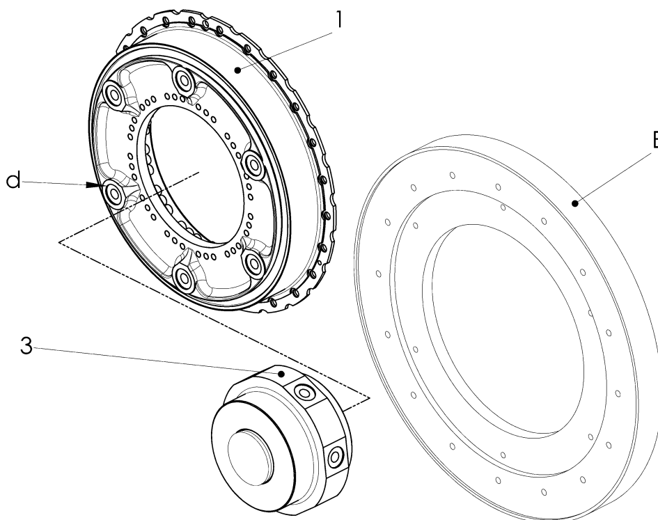
Abbildung 6-5 Baugruppe Lenkerflansch (1) positionieren
