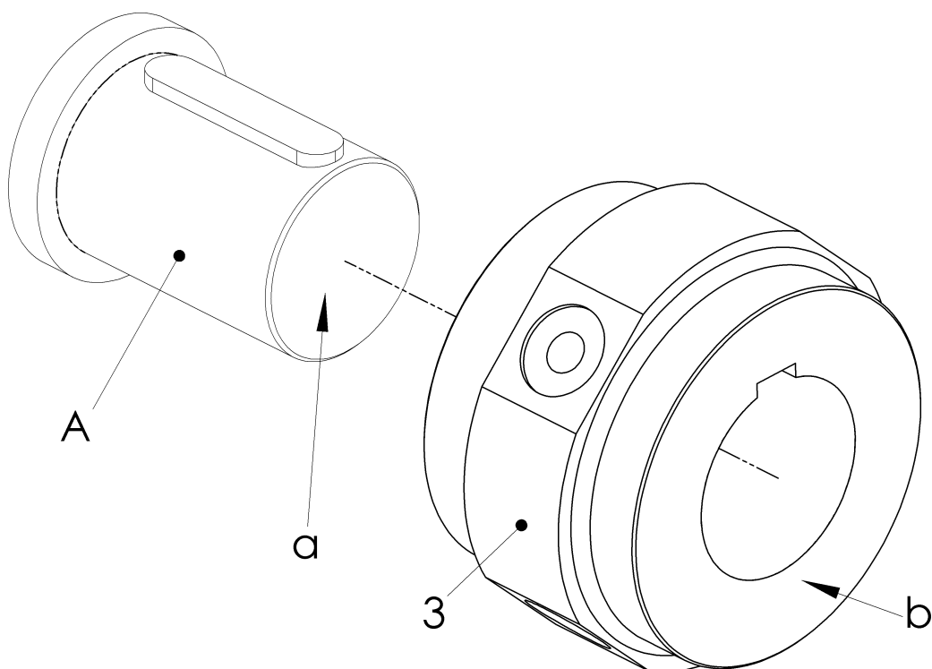
Abbildung 6-3 Nabe mit zylindrischer Bohrung und Passfedernut montieren
