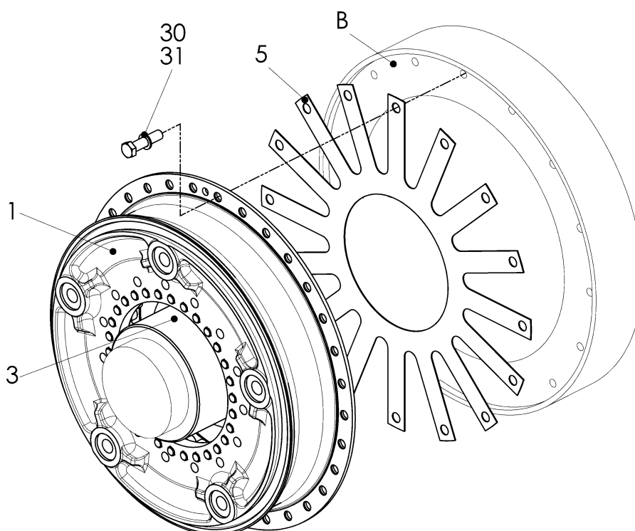
Abbildung 6-6 Baugruppe Lenkerflansch mit/ohne Blech (5) montieren
